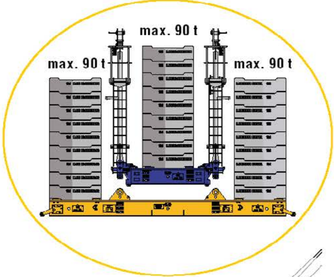
270 t Lisävastapaino alusta 270 t Derrick counterweight optional VarioTray
